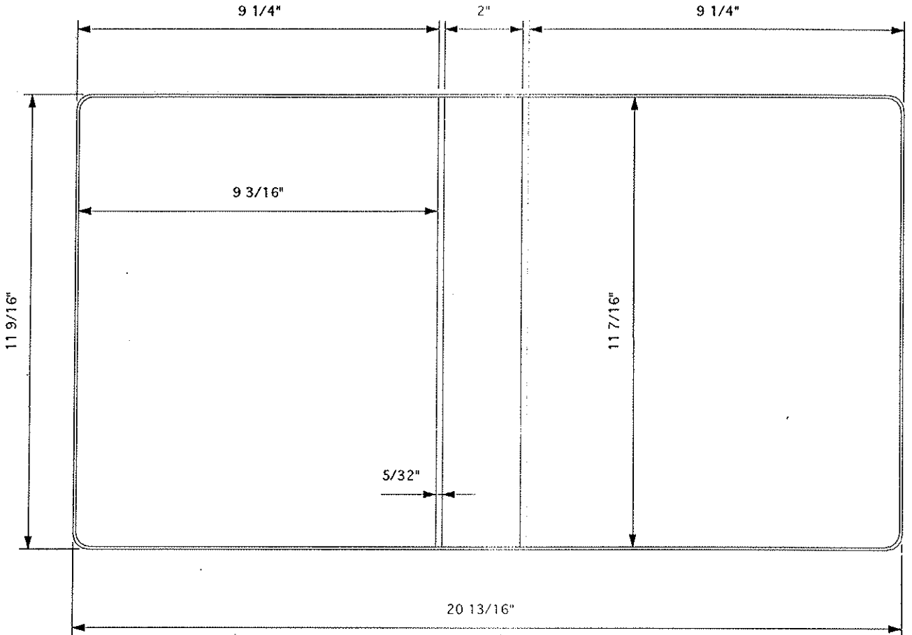
ALUMINUM BASE DIE
